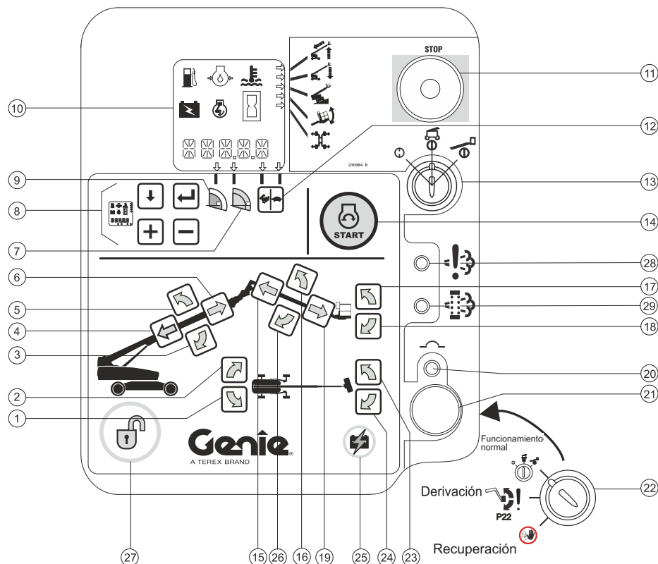
Panel de mandos del suelo
