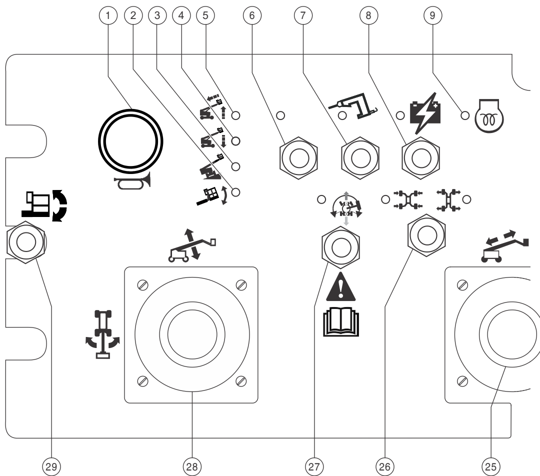
Panel de mandos de la plataforma
